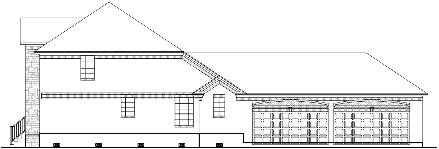
RIGHT ELEVATION
